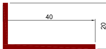
Art.Nr. A8420 Bezeichnung L - Winkelprofil 40x20x2
