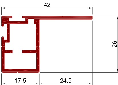
Art.Nr. A1670 Bezeichnung Einbaurahmenprofil Multi mit Falz
