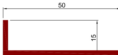
Art.Nr. A8515 Bezeichnung L - Winkelprofil 50x15x2
