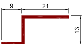
Art.Nr. A7060 Bezeichnung Z - Profil Befestigungsschiene für Spannrahmen
