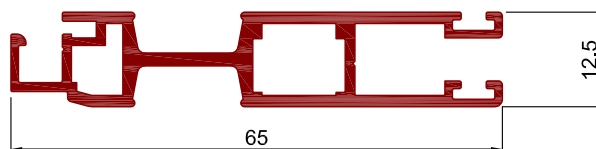
Art.Nr. A1320 Bezeichnung Schieberahmen mit Eingriff
