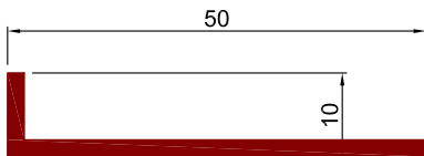
Art.Nr. A8510 Bezeichnung L - Winkelprofil 50x10x2
