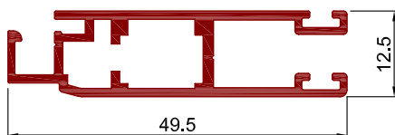
Art.Nr. A1310 Bezeichnung Schieberahmen
