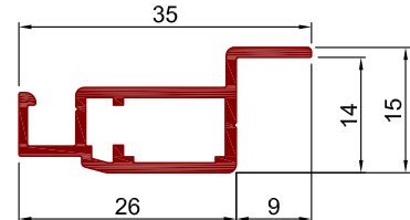
Art.Nr. A1019 Bezeichnung Spannrahmenprofil mit abgesetztem Falz
