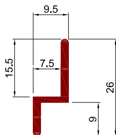
Art.Nr. A1350 Bezeichnung Z - Profil Führungsschiene für Schiebetüre
