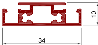
Art.Nr. A1250 Bezeichnung Sprossenprofil gewebeteilend
