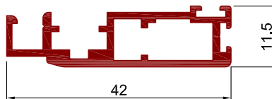
Art.Nr. A1130 Bezeichnung Spannrahmenprofil Typ I mit Bürstenführung
