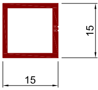
Art.Nr. A1515 Bezeichnung RR - Hohlpr.- Einbaur. 15x15x1.2
