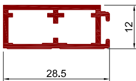
Art.Nr. A2470 Bezeichnung Pendeltür-Einbaurahmenprofil Typ II mit Bürstenführung
