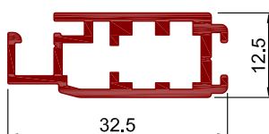
Art.Nr. A1240 Bezeichnung Drehrahmenprofil für Duplextüre
