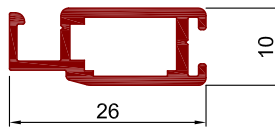
Art.Nr. A1016 Bezeichnung Spannrahmenprofil mit Bürstenführung
