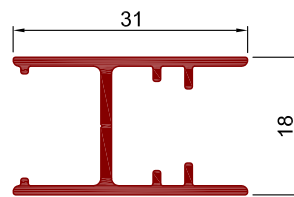
Art.Nr. K2020 Bezeichnung Plissee für Türen Anschlagschiene, seitlich
