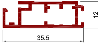
Art.Nr. A2240 Bezeichnung Drehrahmenprofil für Pendeltüre Typ II
