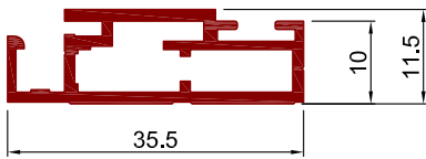
Art.Nr. A2210 Bezeichnung Drehrahmenprofil Typ II
