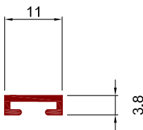
Art.Nr. A7025 Bezeichnung c-Bürstenführungsprofil
