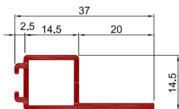
Art.Nr. A1470 Bezeichnung Einbaurahmenprofil mit Falz für Pendeltüren
