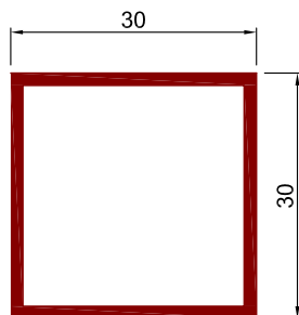
Art.Nr. A9330 Bezeichnung RR - Hohlprofil 30x30x2
