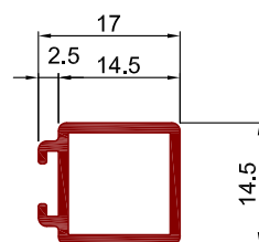
Art.Nr. A1490 Bezeichnung Einbaurahmenprofil für Pendeltüren
