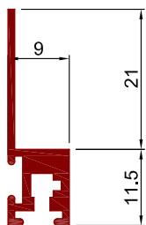
Art.Nr. A7010 Bezeichnung h - Bürstenführungsprofil
