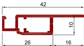
Art.Nr. A1014 Bezeichnung Spannrahmenprofil mit Falz 16 mm
