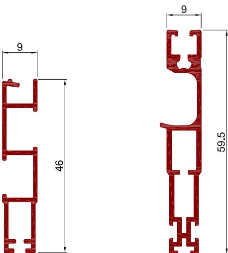
Art.Nr. K1833 Bezeichnung Rollo Zugschiene
