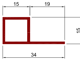
Art.Nr. A1570 Bezeichnung Einbaurahmenprofil
