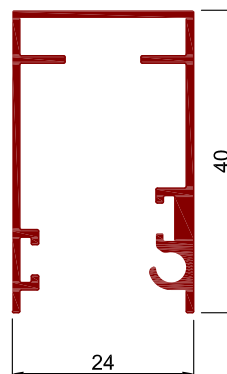
Art.Nr. K1860 Bezeichnung Fenster-/Türrollo-Führungsschiene
