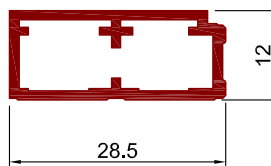
Art.Nr. A2480 Bezeichnung Pendeltür-Einbaurahmenprofil Typ II
