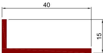
Art.Nr. A8415 Bezeichnung L - Winkelprofil 40x15x2
