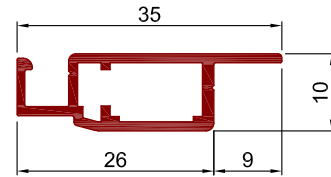
Art.Nr. A1012 Bezeichnung Spannrahmenprofil mit Falz 9 mm
