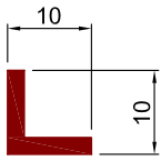
Art.Nr. A8110 Bezeichnung L - Winkelprofil 10x10x2
