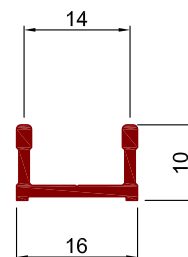
Art.Nr. A1362 Bezeichnung U - Profil Führungsschiene für Schiebetüre
