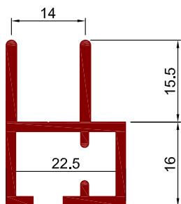
Art.Nr. A1330 Bezeichnung Einbaurahmenprofil für Schiebetüre
