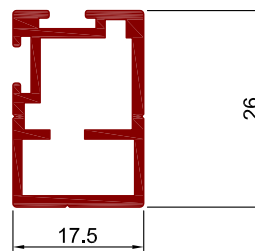
Art.Nr. A1690 Bezeichnung Einbaurahmenprofil Multi
