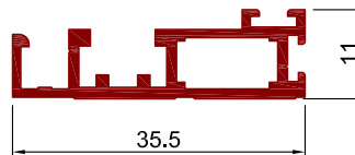
Art.Nr. A2116 Bezeichnung Spannrahmenprofil Typ II mit Bürstenführungen
