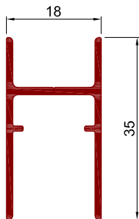
Art.Nr. K2030 Bezeichnung Plissee Führungsschiene, oben
