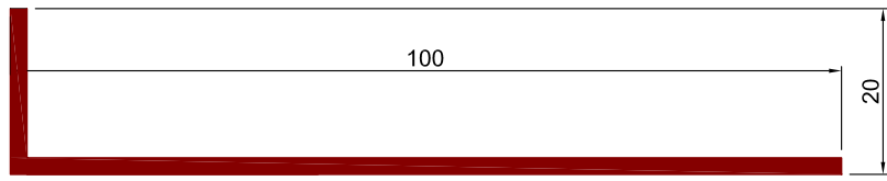
Art.Nr. A8120 Bezeichnung L - Winkelprofil 100x20x2
