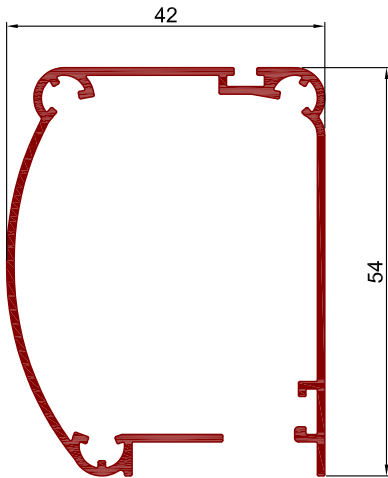
Art.Nr. K1831 Bezeichnung Rollokassette
