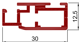
Art.Nr. A1210 Bezeichnung Drehrahmenprofil
