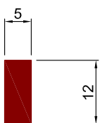
Art.Nr. A9112 Bezeichnung FL - Flachprofil 12x5
