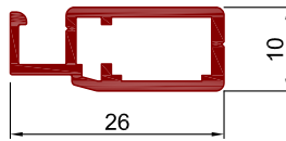
Art.Nr. A1010 Bezeichnung Spannrahmenprofil
