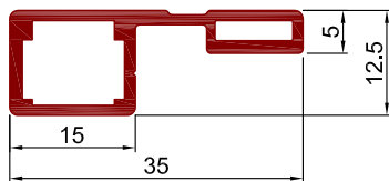
Art.Nr. A1280 Bezeichnung Einbaurahmenprofil
