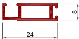
Art.Nr. A2008 Bezeichnung Spannrahmenprofil 8 mm
