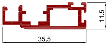
Art.Nr. A1120 Bezeichnung Spannrahmenprofil Typ I mit Bürstenführung
